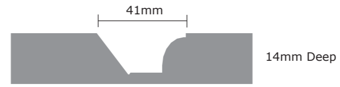
Door Profile
